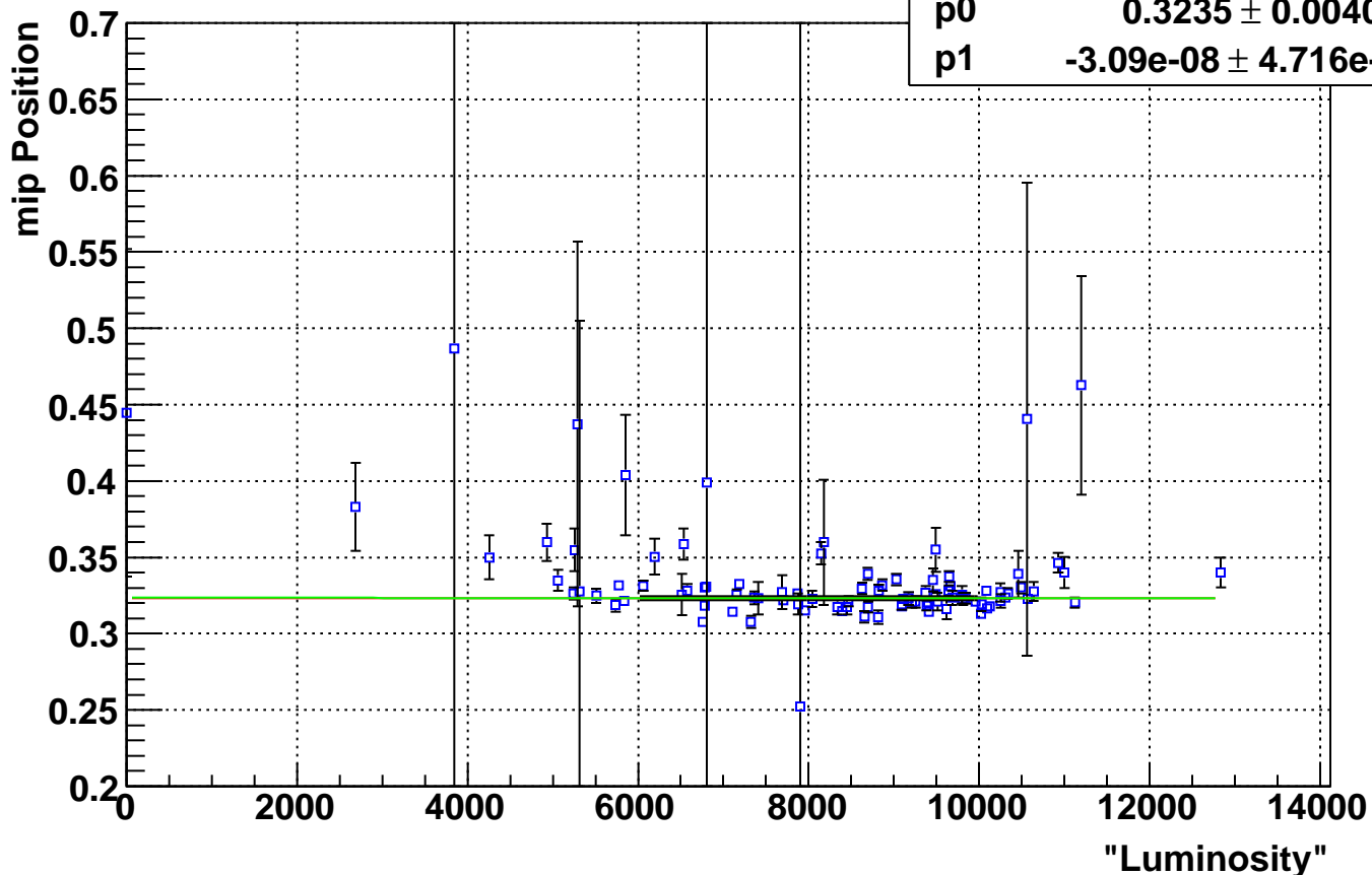
Eta Bin 36 mip Positons Vs. Luminosity
