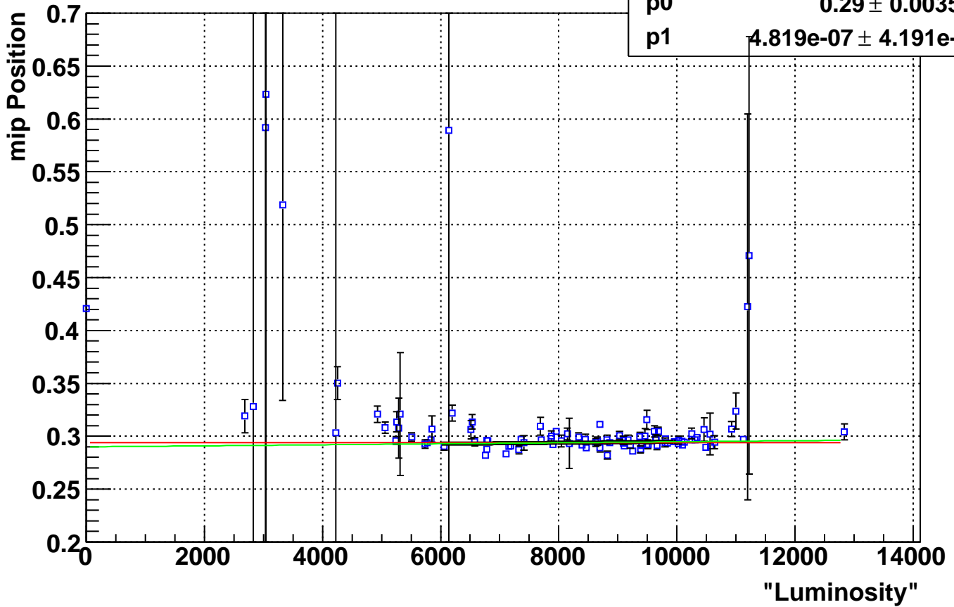
Eta Bin 10 mip Positons Vs. Luminosity
