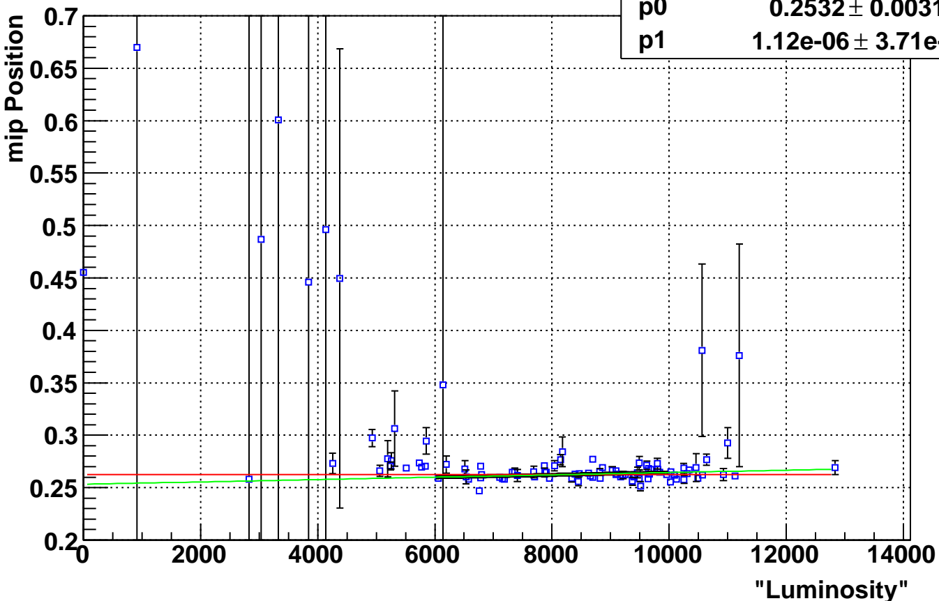
Eta Bin 14 mip Positons Vs. Luminosity
