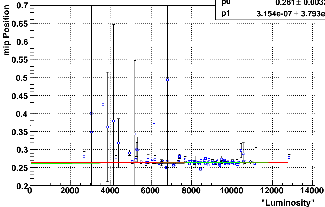
Eta Bin 28 mip Positons Vs. Luminosity
