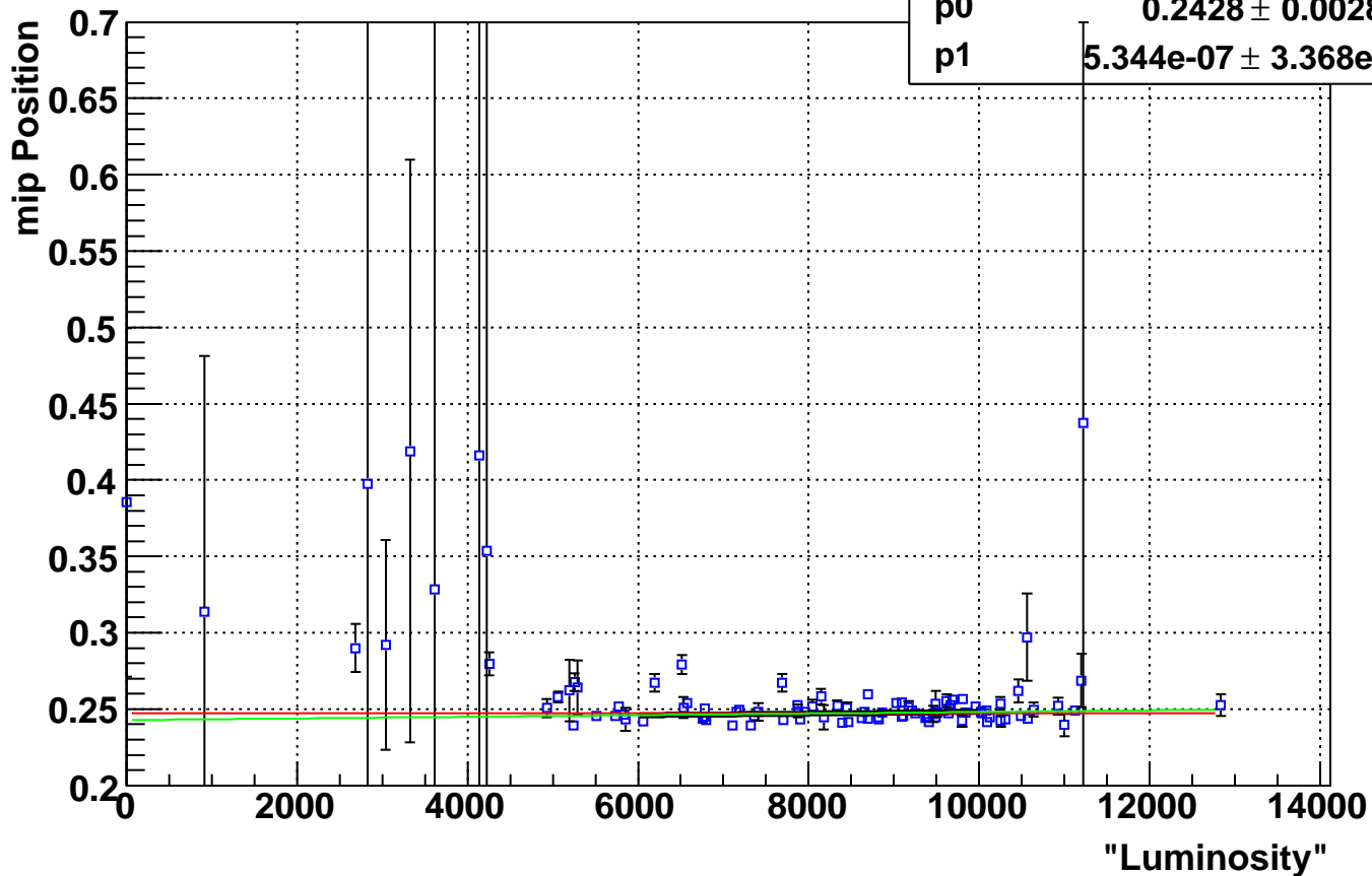
Eta Bin 18 mip Positons Vs. Luminosity
