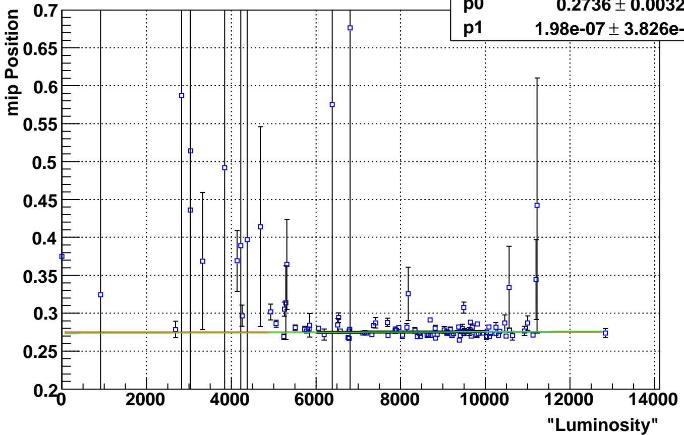
Eta Bin 12 mip Positons Vs. Luminosity
