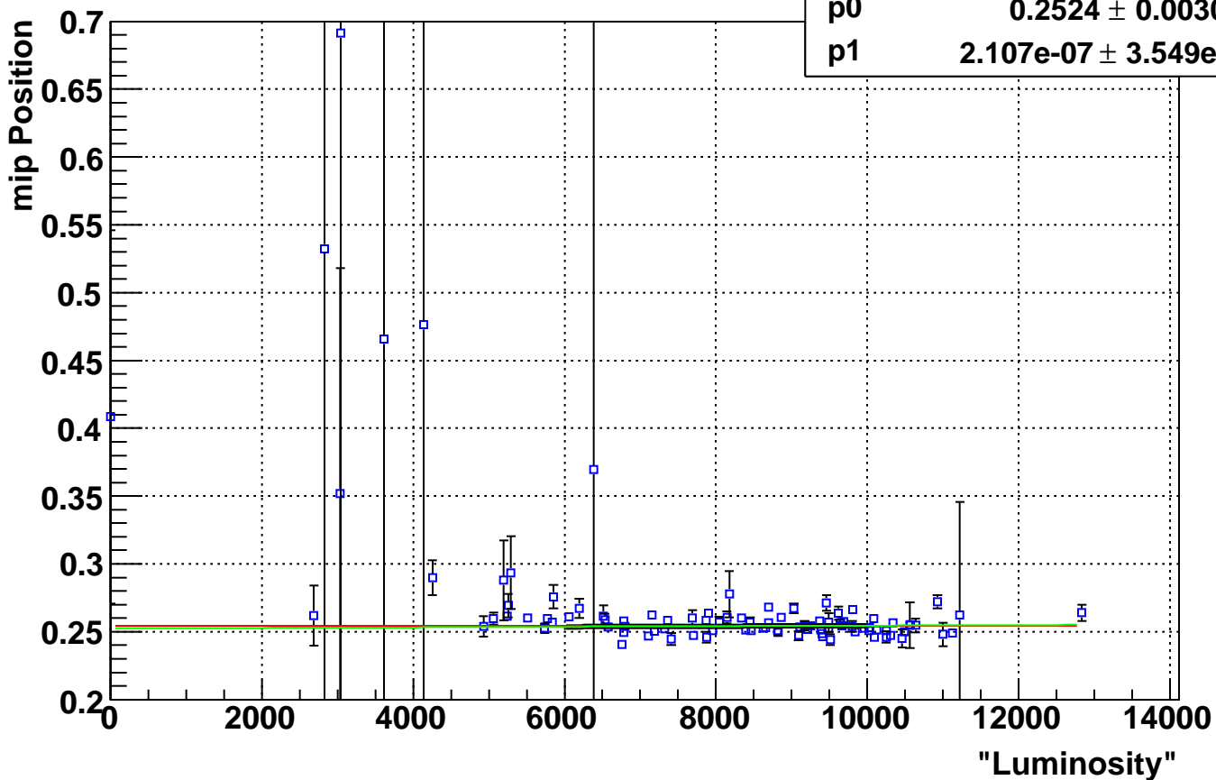
Eta Bin 16 mip Positons Vs. Luminosity
