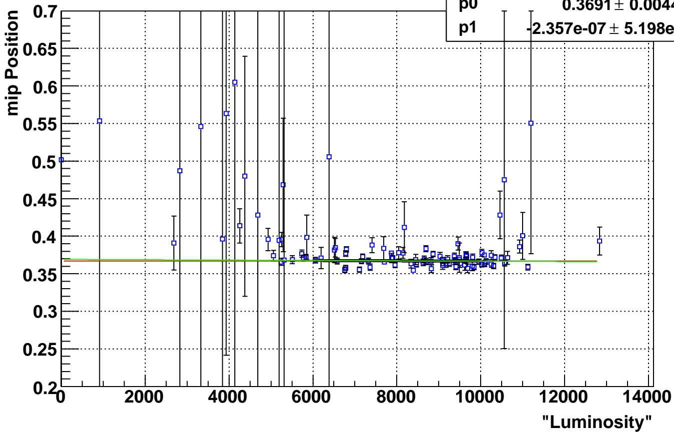
Eta Bin 38 mip Positons Vs. Luminosity
