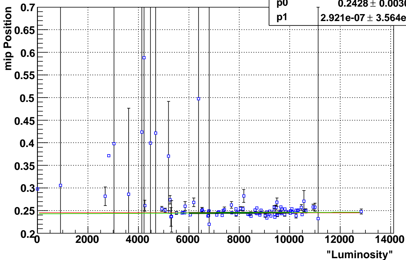
Eta Bin 22 mip Positons Vs. Luminosity
