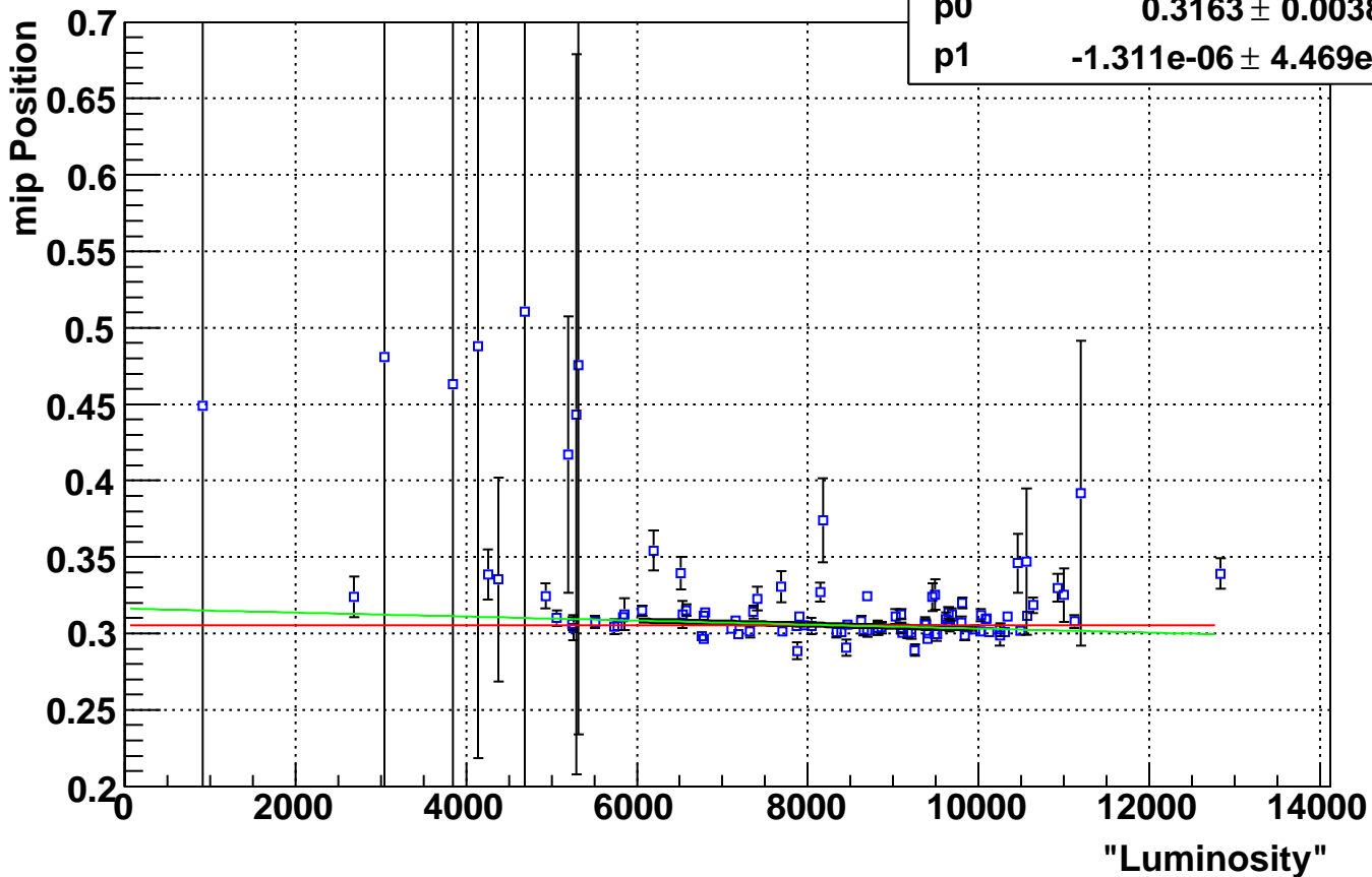
Eta Bin 8 mip Positons Vs. Luminosity
