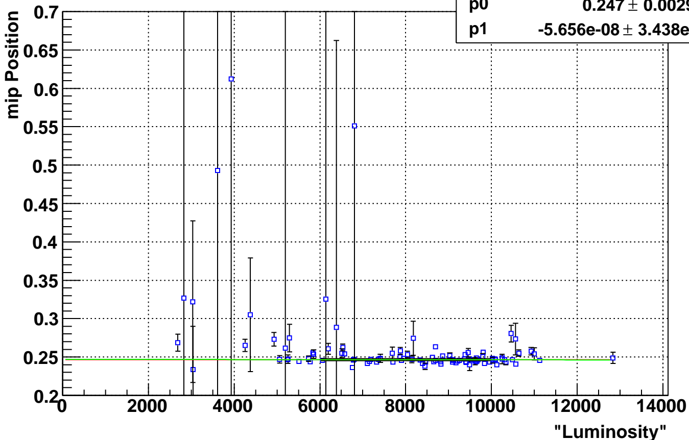
Eta Bin 20 mip Positons Vs. Luminosity
