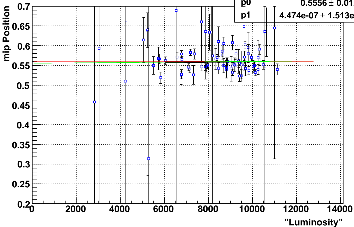
Eta Bin 40 mip Positons Vs. Luminosity
