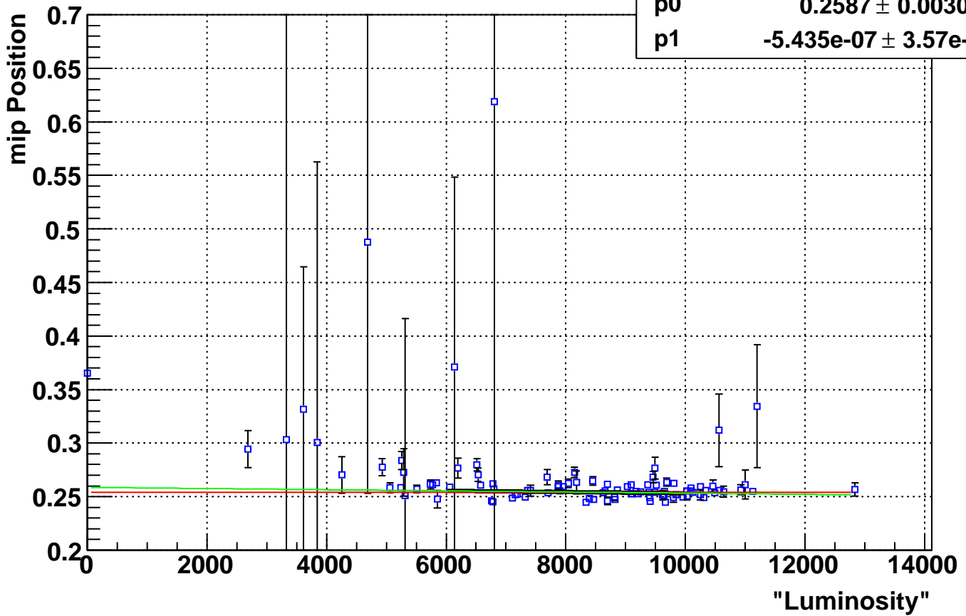
Eta Bin 26 mip Positons Vs. Luminosity
