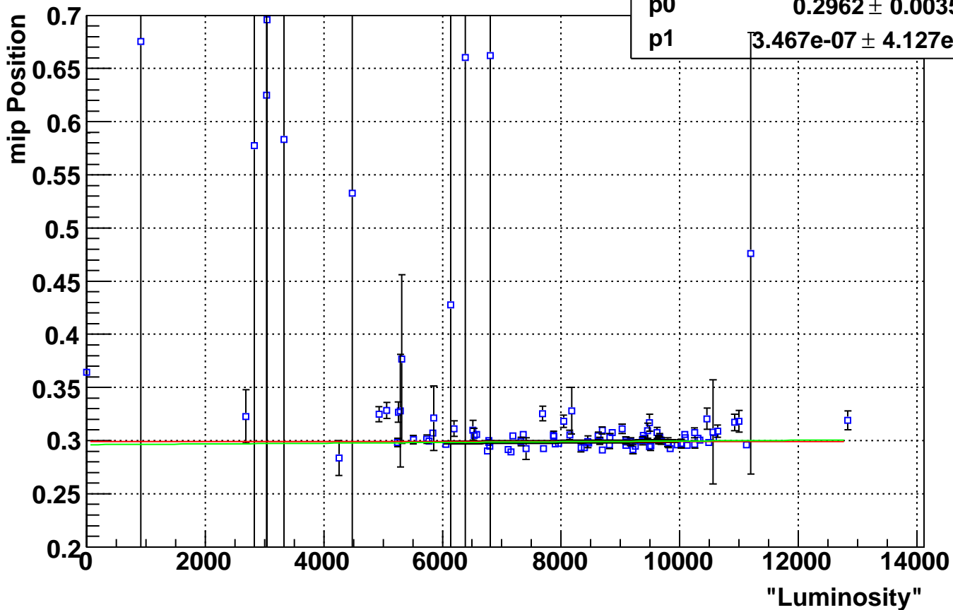
Eta Bin 32 mip Positons Vs. Luminosity
