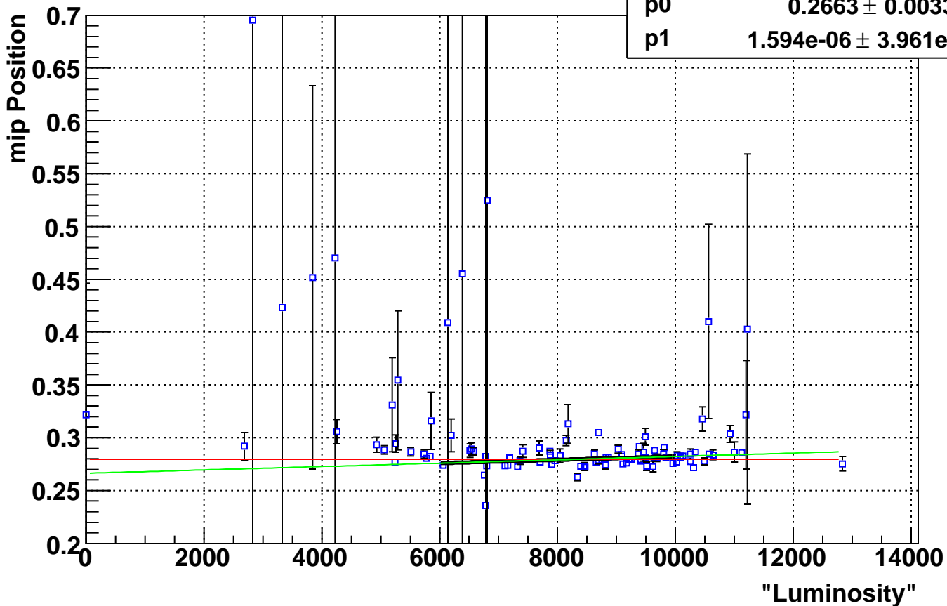
Eta Bin 30 mip Positons Vs. Luminosity
