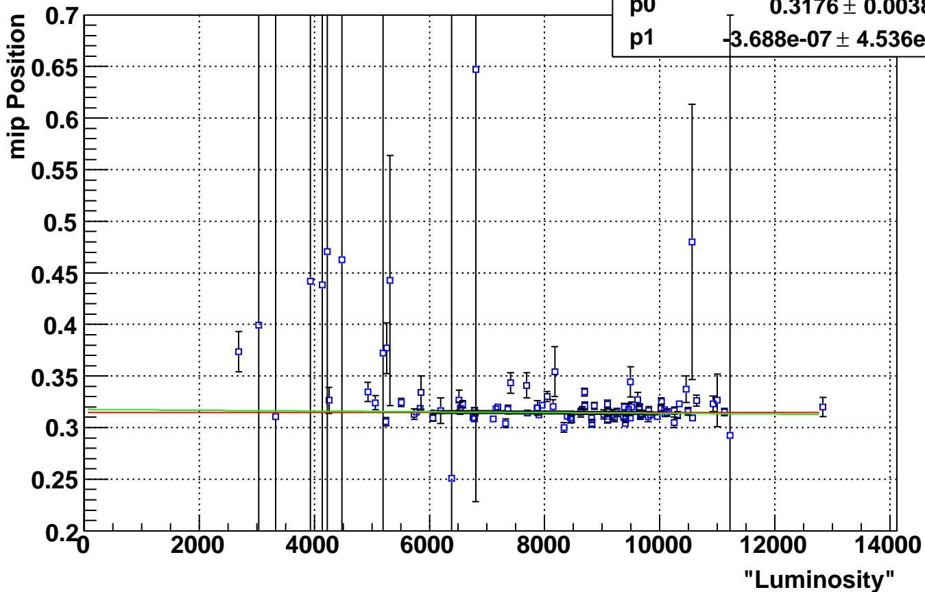
Eta Bin 34 mip Positons Vs. Luminosity
