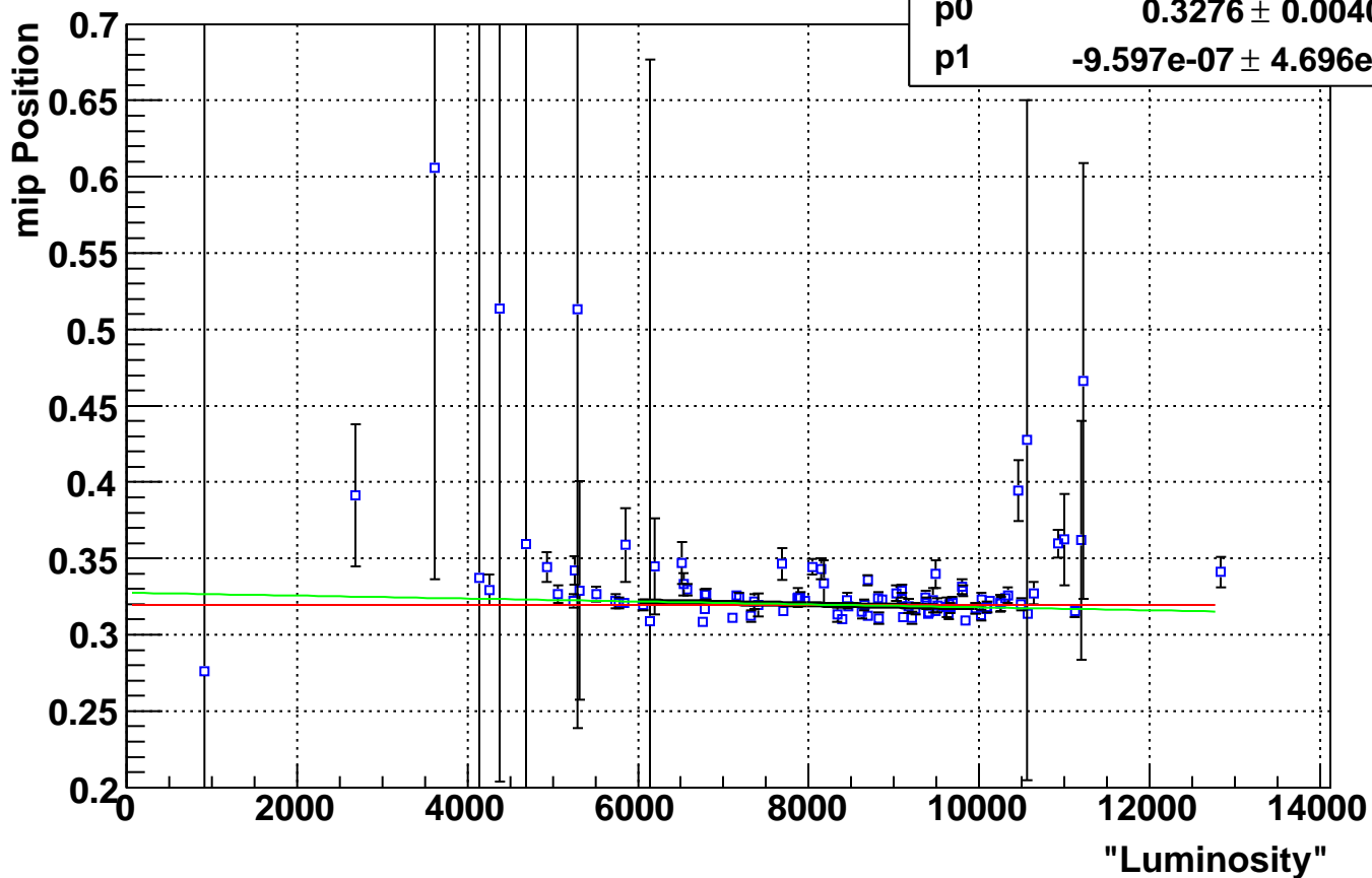
Eta Bin 6 mip Positons Vs. Luminosity
