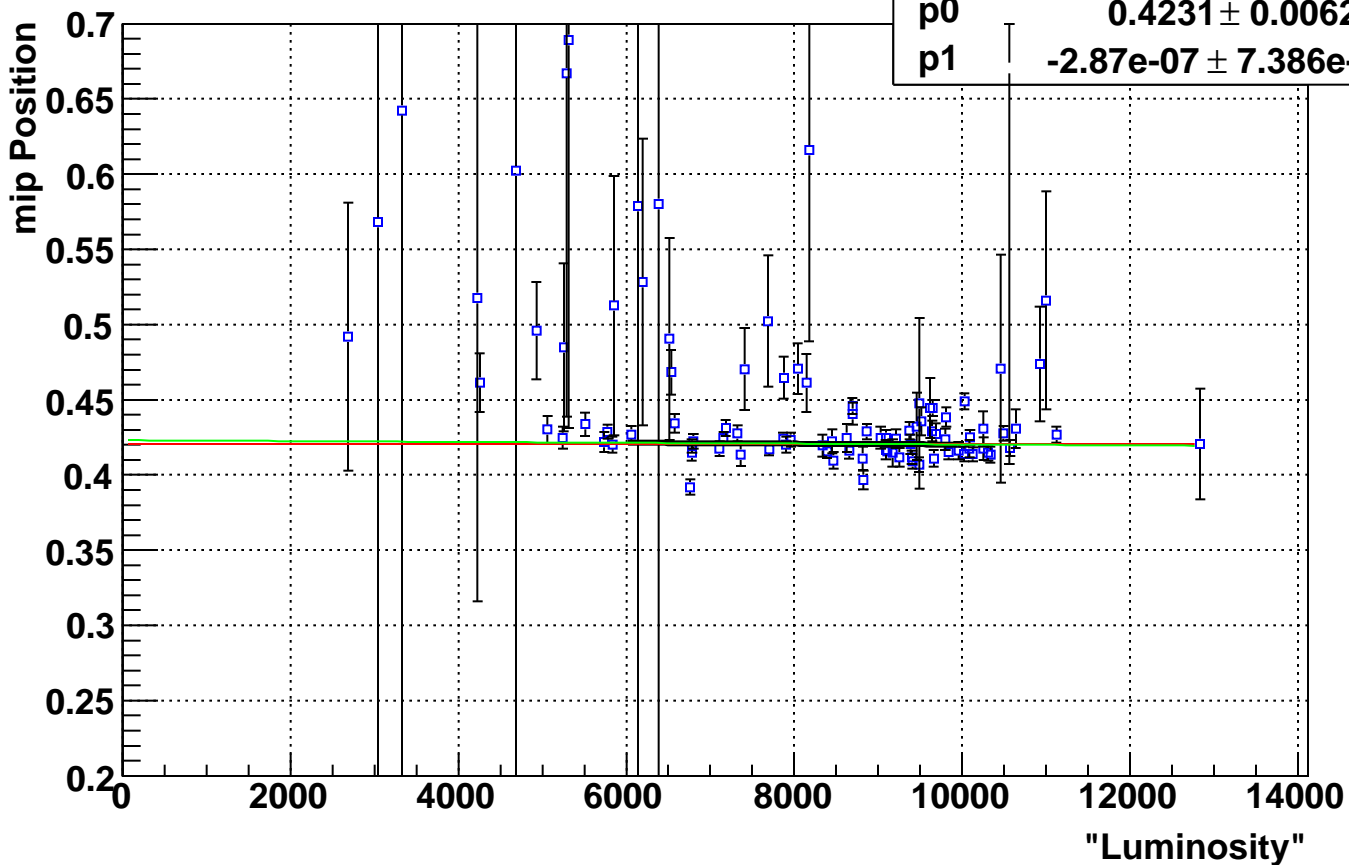
Eta Bin 2 mip Positons Vs. Luminosity
