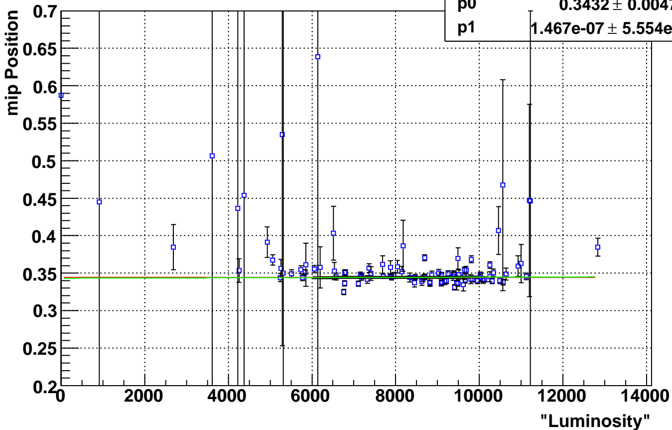
Eta Bin 4 mip Positons Vs. Luminosity
