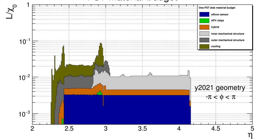
FST Material Budget
