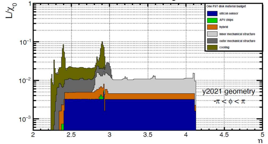
FST Material Budget
