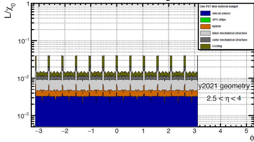
FST Material Budget
