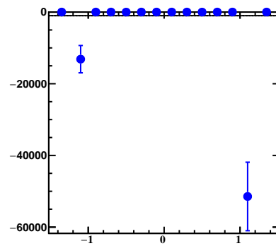
Cent 4 0.0<pT<0.0 y
