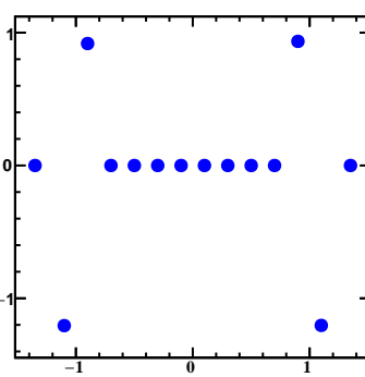
Cent 4 0.0<pT<0.0 y
