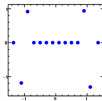
Cent 4 0.0<pT<0.0 y
