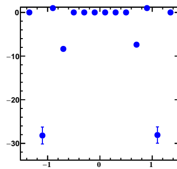
Cent 4 0.0<pT<0.0 y
