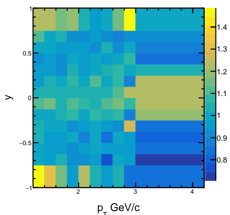
Data/Embedding
