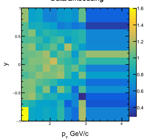
Data/Embedding
