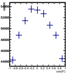
Raw Yields 0/5 < y < 1/5
