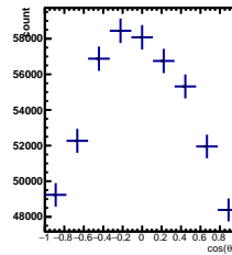
Raw Yields -2/5 < y < -1/5
