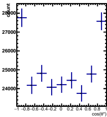
Raw Yields -4/5 < y < -3/5
