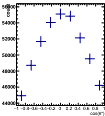
Raw Yields 1/5 < y < 2/5
