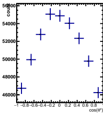
Raw Yields -1/5 < y < 0/5
