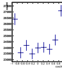
Raw Yields 3/5 < y < 4/5
