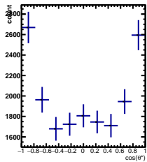
Raw Yields -5/5 < y < -4/5
