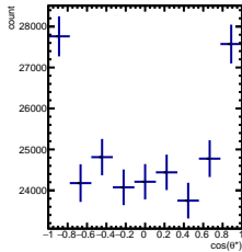
Raw Yields -4/5 < y < -3/5
