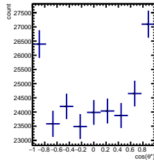
Raw Yields 3/5 < y < 4/5
