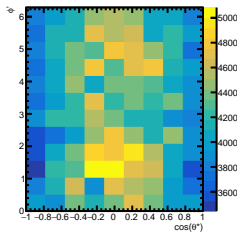
Raw Yields 1/5 < y < 2/5
