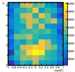
Raw Yields 0/5 < y < 1/5
