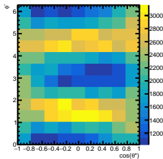
Raw Yields 3/5 < y < 4/5
