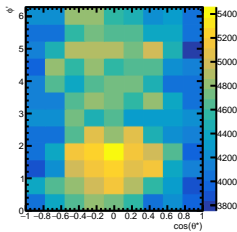
Raw Yields -2/5 < y < -1/5
