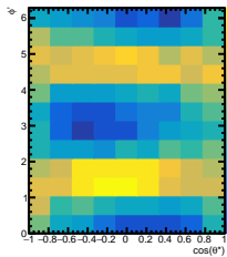
Raw Yields -4/5 < y < -3/5
