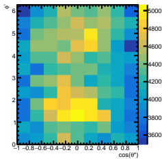
Raw Yields -1/5 < y < 0/5
