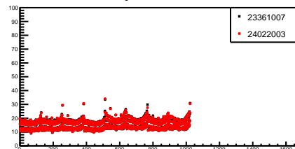
g_ranStdDev_19_1
