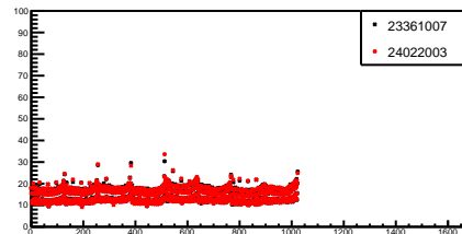
g_ranStdDev_7_0
