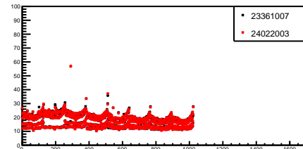
g_ranStdDev_6_1
