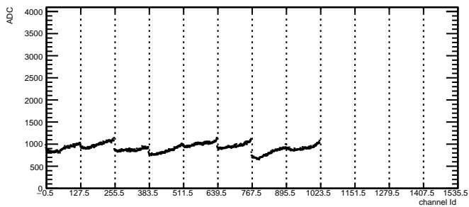
Pedestal: RDO2 Module9 TB2
