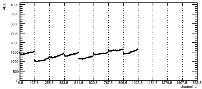
Pedestal: RDO3 Module3 TB1
