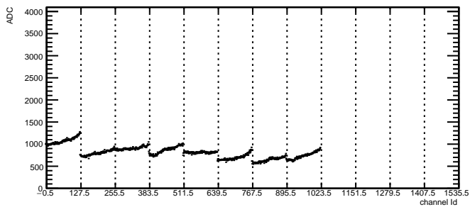
Pedestal: RDO5 Module3 TB1
