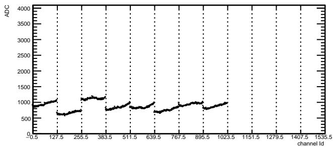
Pedestal: RDO4 Module10 TB0
