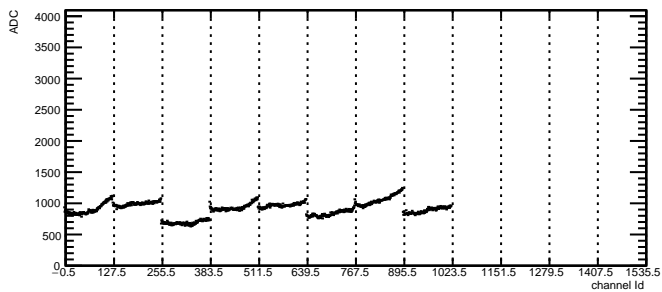
Pedestal: RDO4 Module9 TB0
