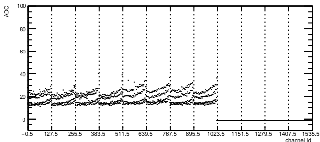
Total Noise: RDO4 Module11 TB0
