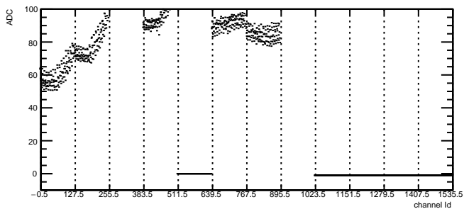
Total Noise: RDO6 Module7 TB0
