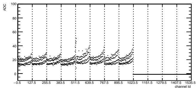
Total Noise: RDO2 Module12 TB1
