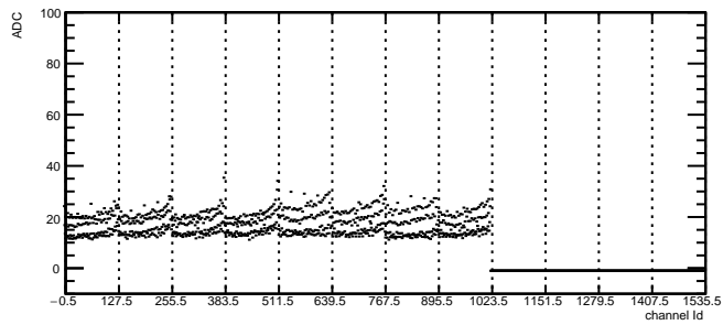
Total Noise: RDO2 Module10 TB0
