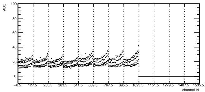
Total Noise: RDO4 Module7 TB1
