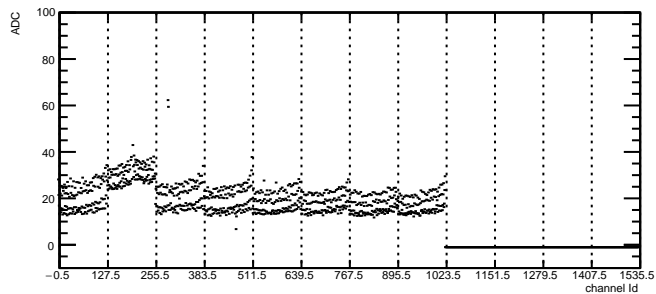
Total Noise: RDO1 Module6 TB2
