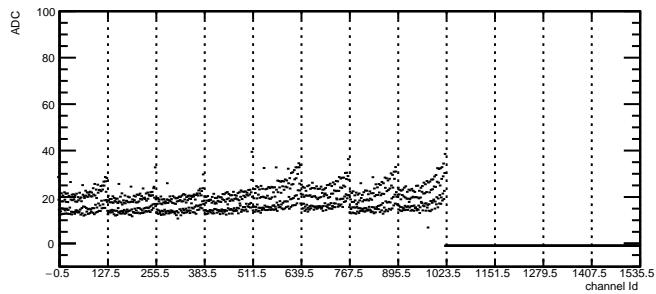
Total Noise: RDO3 Module4 TB0
