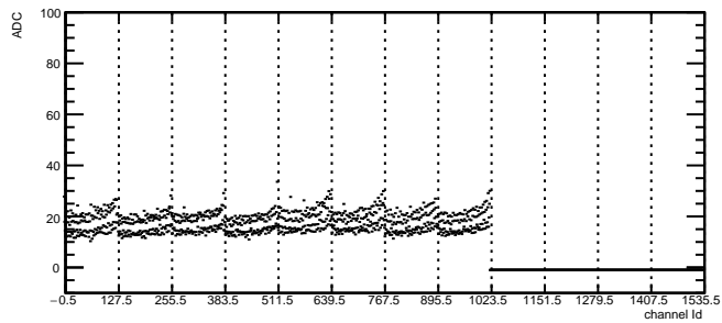
Total Noise: RDO4 Module10 TB2
