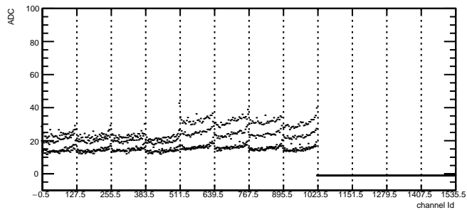
Total Noise: RDO1 Module2 TB2
