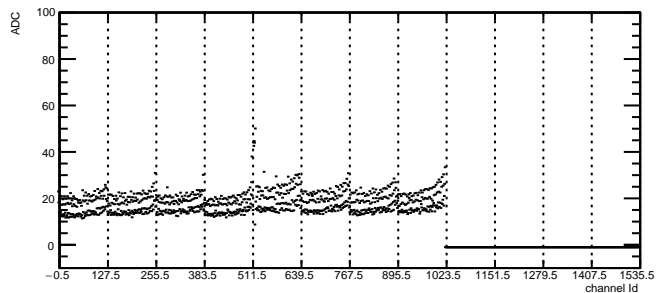
Total Noise: RDO2 Module12 TB2
