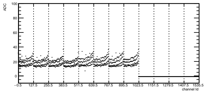
Total Noise: RDO1 Module4 TB0
