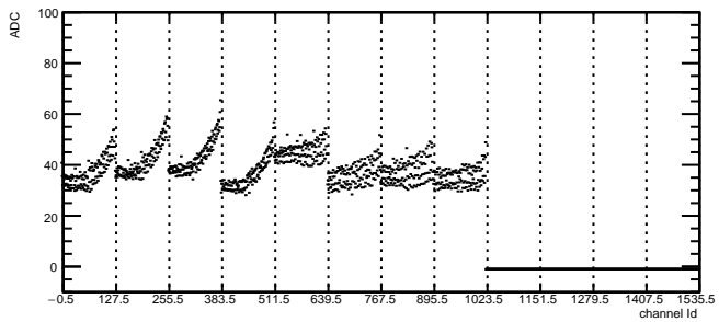
Total Noise: RDO5 Module3 TB1
