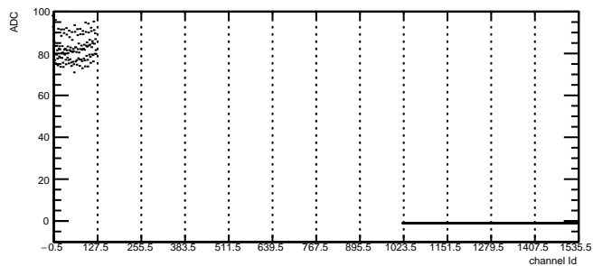
Total Noise: RDO6 Module8 TB0
