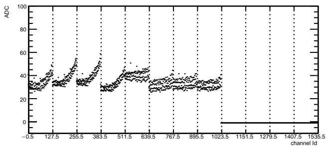
Total Noise: RDO5 Module3 TB2
