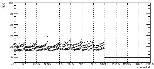
Total Noise: RDO2 Module10 TB1
