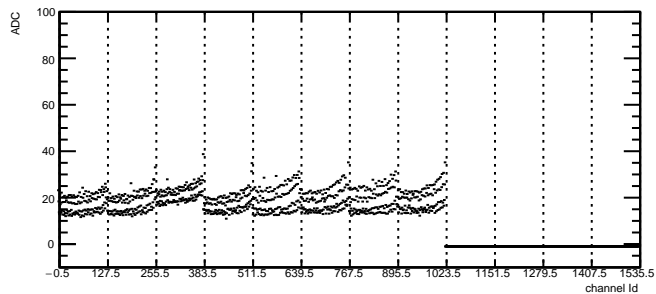
Total Noise: RDO4 Module8 TB0
