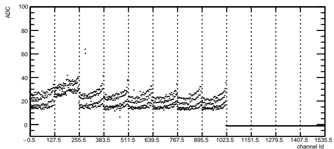
Total Noise: RDO1 Module6 TB1
