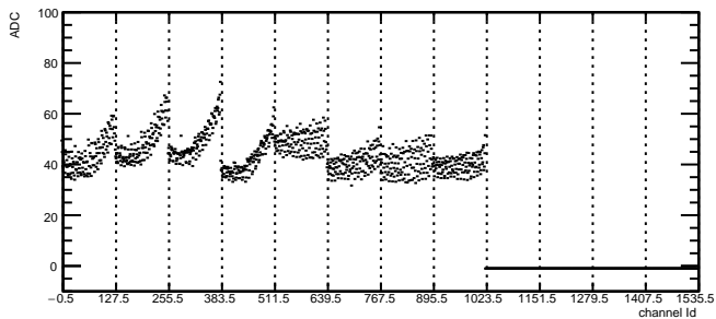
Total Noise: RDO5 Module3 TB0
