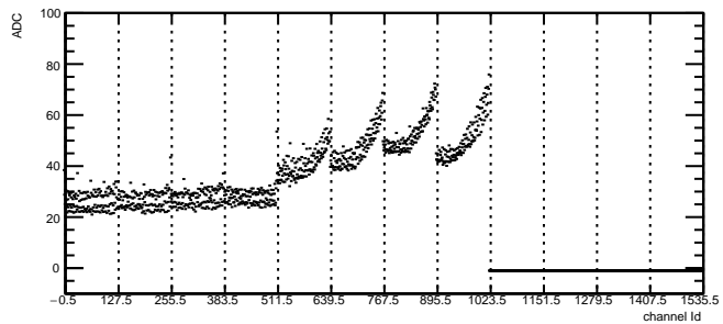
Total Noise: RDO5 Module2 TB1
