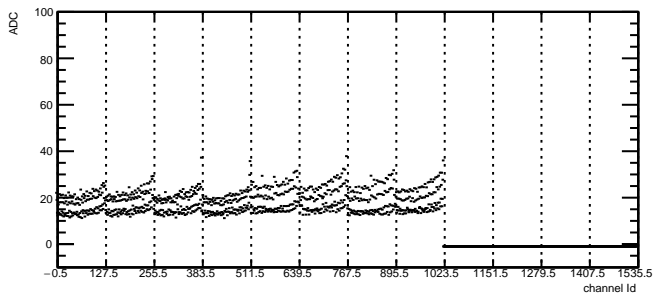
Total Noise: RDO4 Module7 TB0
