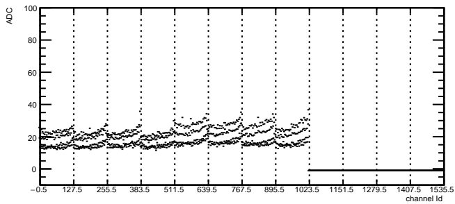
Total Noise: RDO3 Module3 TB0
