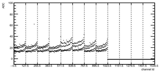
Total Noise: RDO3 Module1 TB1
