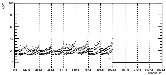
Total Noise: RDO2 Module9 TB1
