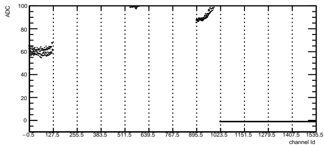
Total Noise: RDO6 Module8 TB2
