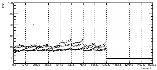
Total Noise: RDO3 Module1 TB2
