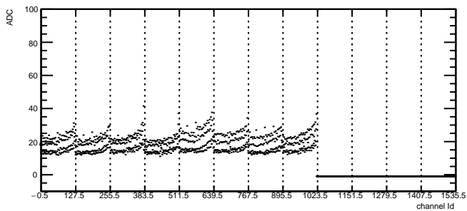
Total Noise: RDO2 Module7 TB1
