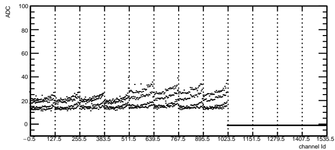
Total Noise: RDO3 Module2 TB0
