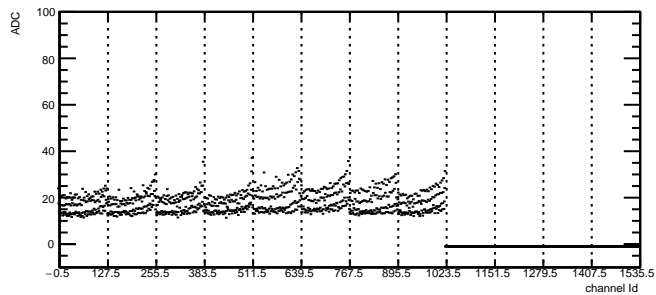
Total Noise: RDO2 Module8 TB0
