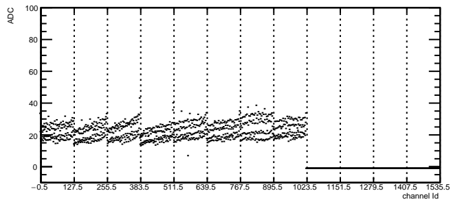
Total Noise: RDO1 Module4 TB2
