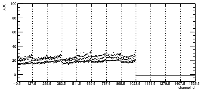
Total Noise: RDO2 Module11 TB2
