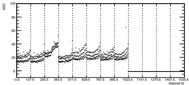
Total Noise: RDO1 Module5 TB0
