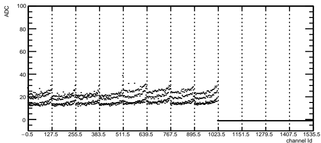
Total Noise: RDO4 Module11 TB2
