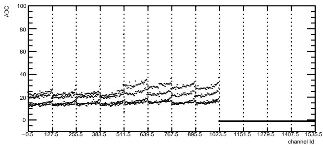
Total Noise: RDO1 Module1 TB2
