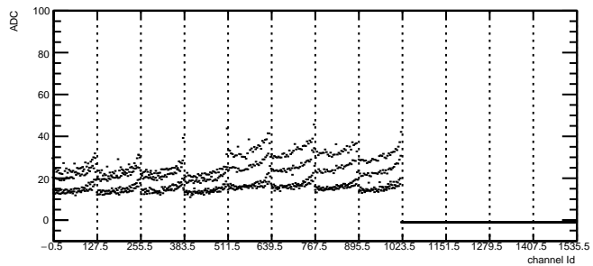
Total Noise: RDO1 Module2 TB1
