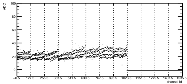
Total Noise: RDO3 Module4 TB2
