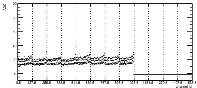
Total Noise: RDO3 Module6 TB2
