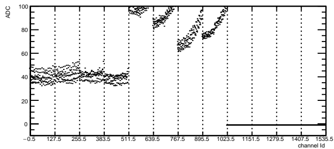
Total Noise: RDO6 Module10 TB0
