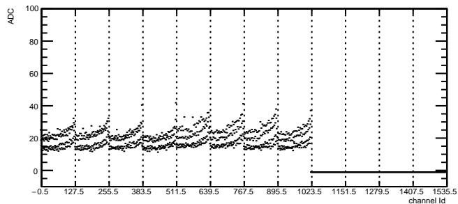
Total Noise: RDO4 Module12 TB1
