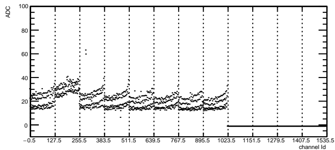
Total Noise: RDO1 Module6 TB0
