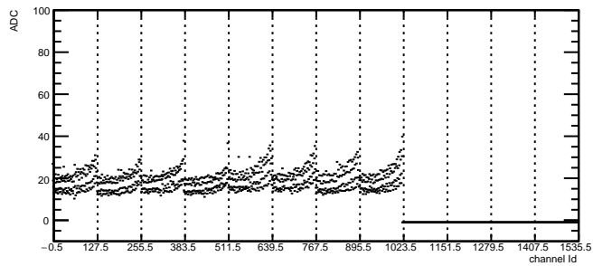
Total Noise: RDO4 Module10 TB1
