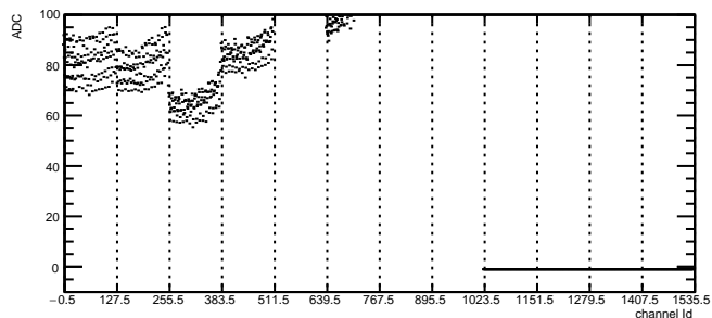
Total Noise: RDO6 Module12 TB0
