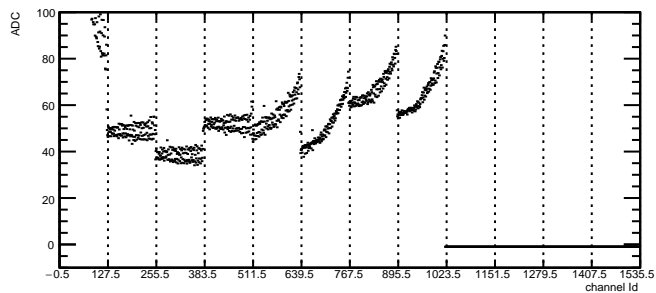
Total Noise: RDO5 Module4 TB2
