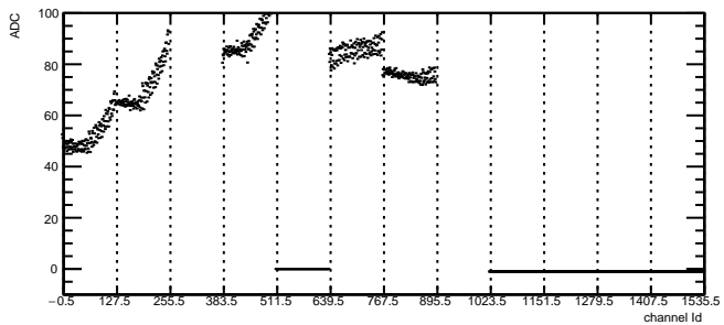
Total Noise: RDO6 Module7 TB1
