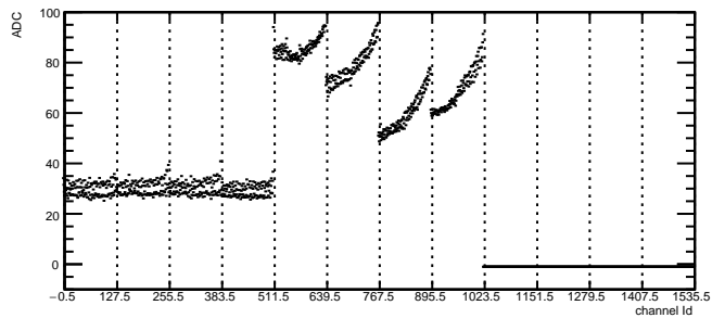
Total Noise: RDO6 Module10 TB2
