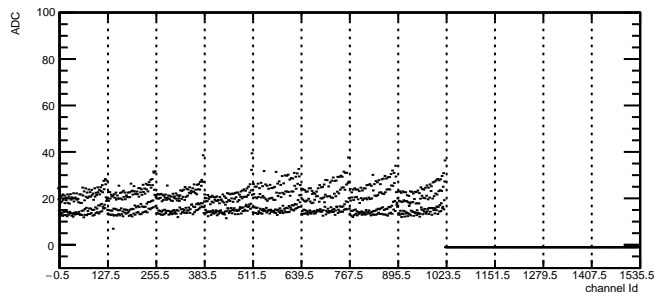
Total Noise: RDO4 Module12 TB0
