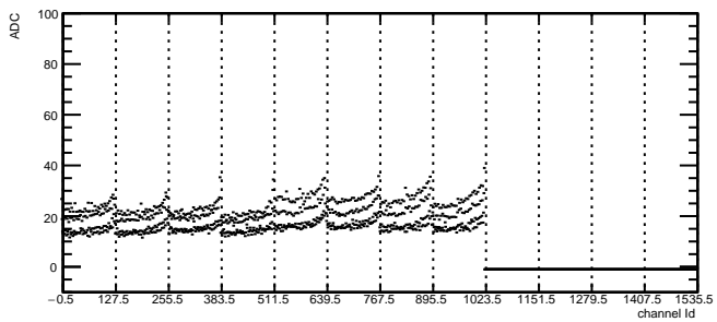
Total Noise: RDO3 Module3 TB1
