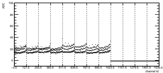
Total Noise: RDO2 Module7 TB2
