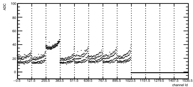
Total Noise: RDO4 Module8 TB1
