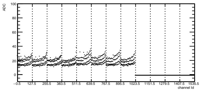
Total Noise: RDO1 Module3 TB1
