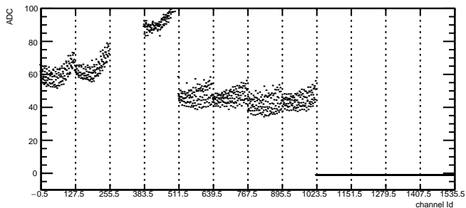
Total Noise: RDO5 Module1 TB0
