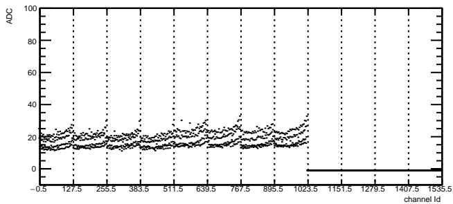
Total Noise: RDO4 Module7 TB2
