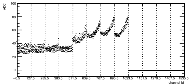
Total Noise: RDO5 Module2 TB0
