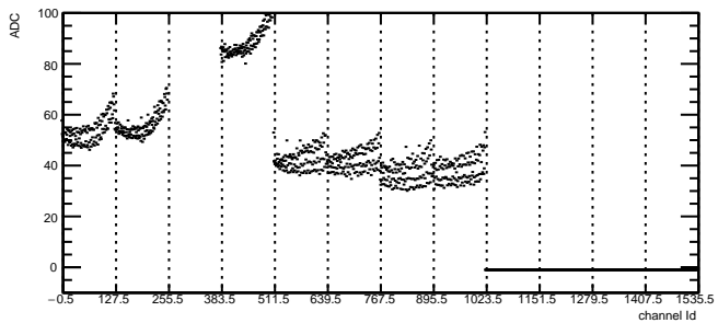
Total Noise: RDO5 Module1 TB1
