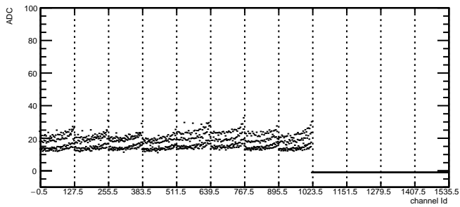
Total Noise: RDO1 Module3 TB2
