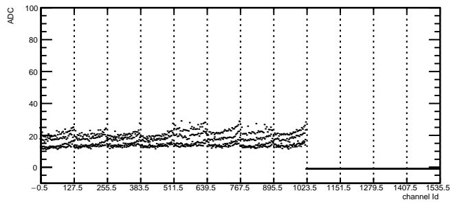
Total Noise: RDO2 Module10 TB2
