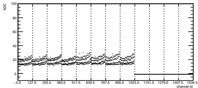
Total Noise: RDO3 Module6 TB0
