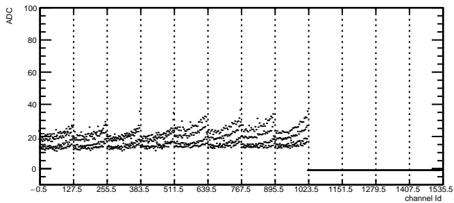
Total Noise: RDO4 Module9 TB0
