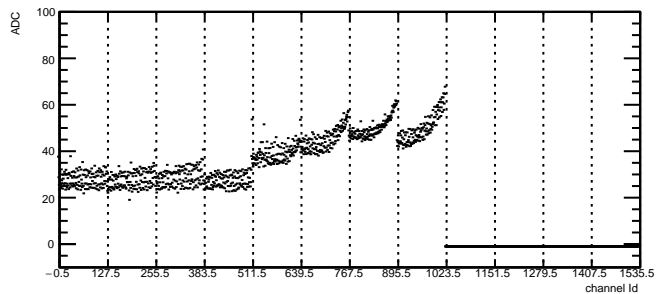
Total Noise: RDO5 Module2 TB2
