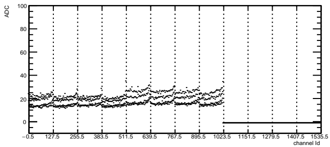
Total Noise: RDO3 Module3 TB2
