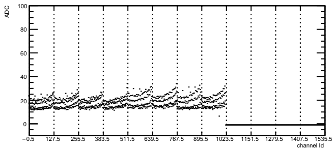
Total Noise: RDO2 Module9 TB0
