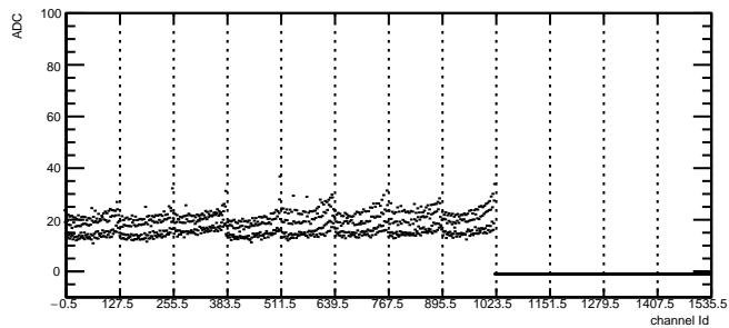
Total Noise: RDO4 Module8 TB2
