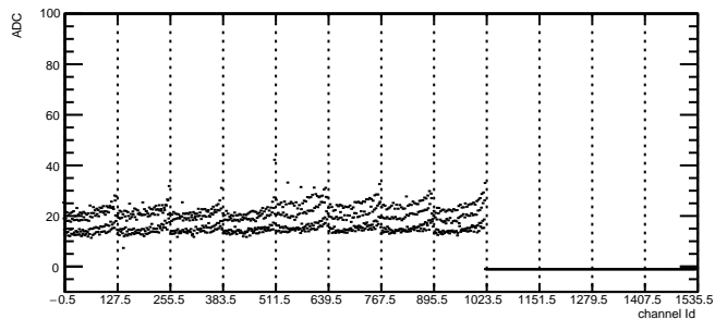
Total Noise: RDO4 Module12 TB2
