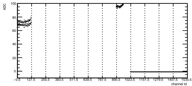
Total Noise: RDO6 Module8 TB1
