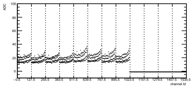
Total Noise: RDO2 Module8 TB1
