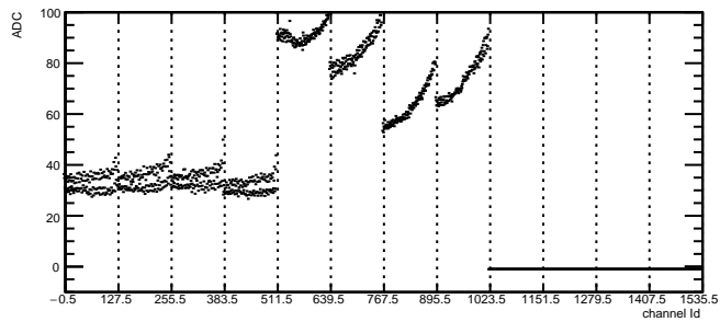
Total Noise: RDO6 Module10 TB1
