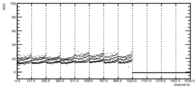
Total Noise: RDO2 Module9 TB2
