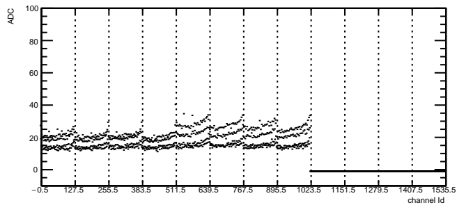
Total Noise: RDO3 Module2 TB2
