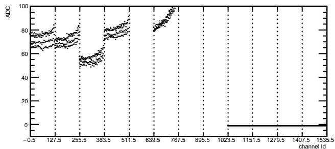
Total Noise: RDO6 Module12 TB1
