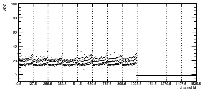
Total Noise: RDO1 Module4 TB1
