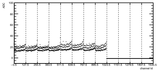
Total Noise: RDO2 Module8 TB2
