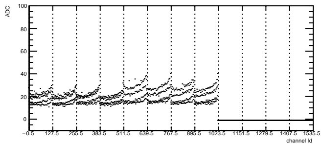
Total Noise: RDO3 Module2 TB1
