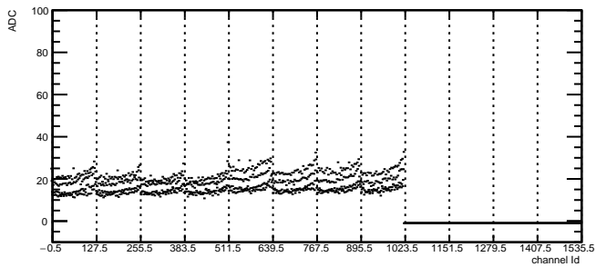
Total Noise: RDO4 Module9 TB2
