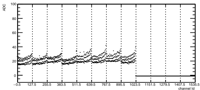
Total Noise: RDO2 Module11 TB1
