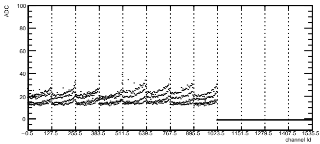
Total Noise: RDO1 Module3 TB0
