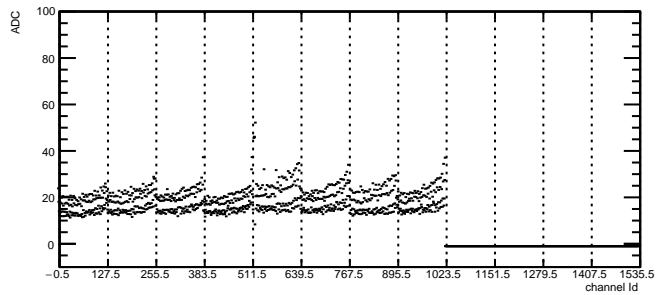
Total Noise: RDO2 Module12 TB0
