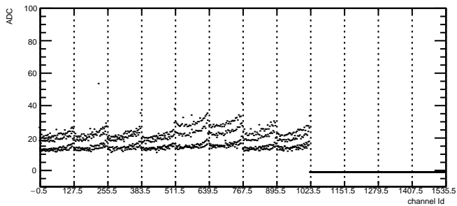
Total Noise: RDO3 Module1 TB0
