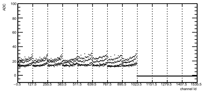
Total Noise: RDO2 Module7 TB0
