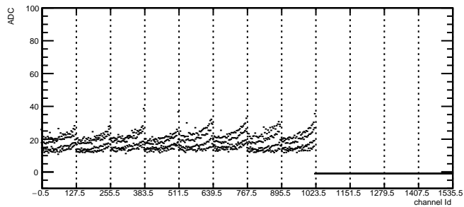
Total Noise: RDO4 Module10 TB0
