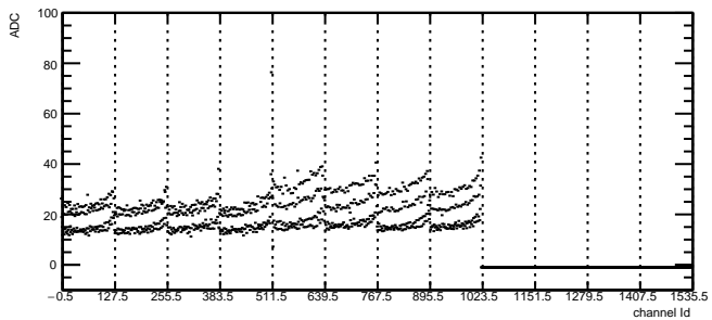
Total Noise: RDO1 Module1 TB1
